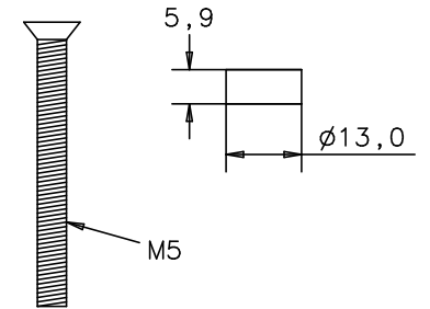
Seitenansichten side views
