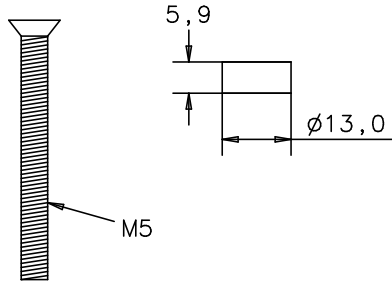
Vorderansicht / Rückansicht front view / back view
