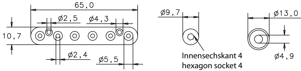
Draufsicht top view
