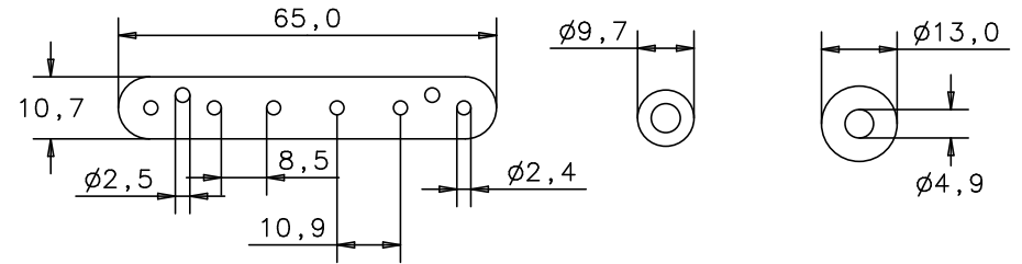
Untersicht bottom view
